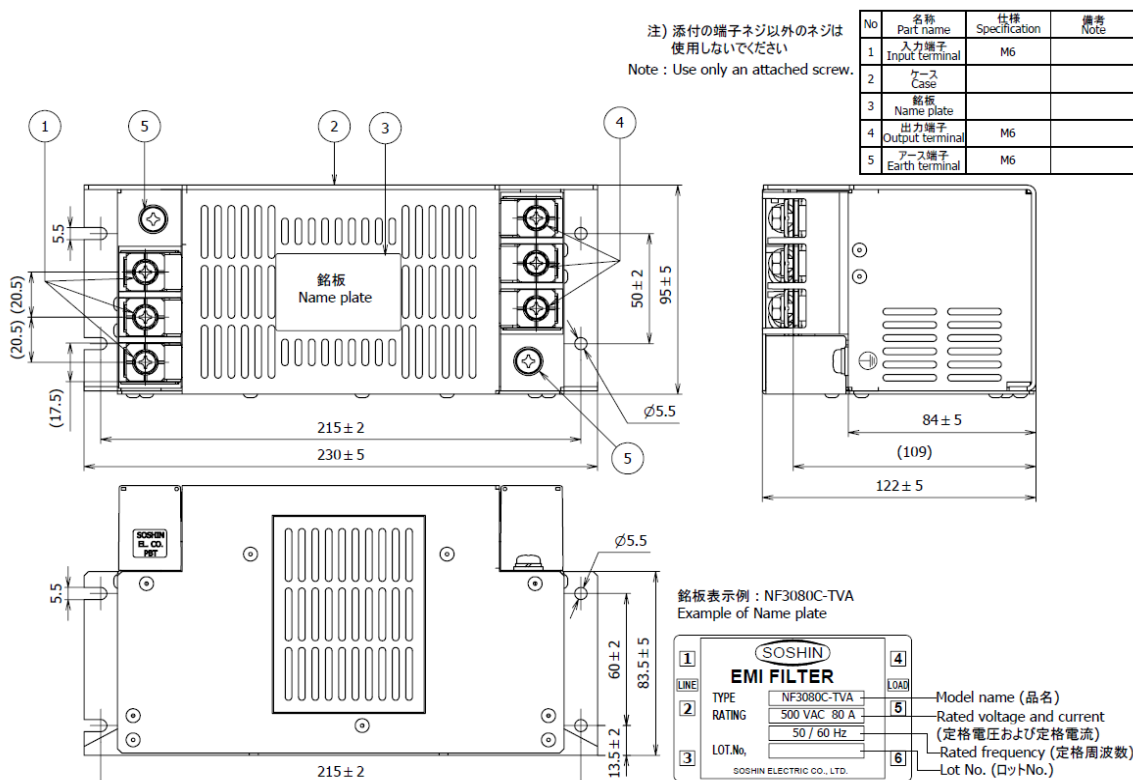
fig.1 (80~100A)
