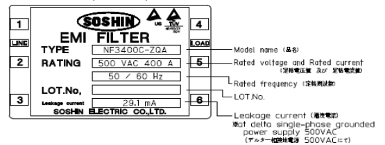
銘板表示例 Example of Name plate
