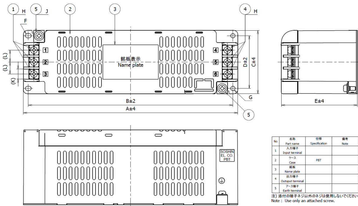
fig.1 (10~60A)
