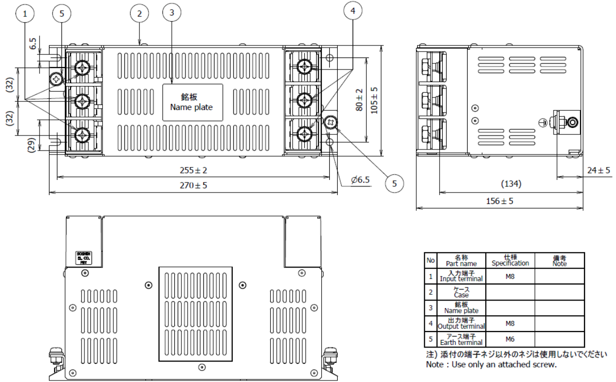
fig. 4 (150~180A)
