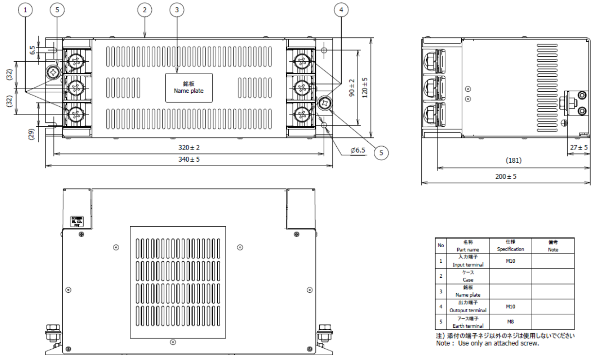
fig. 5 (200~300A)
