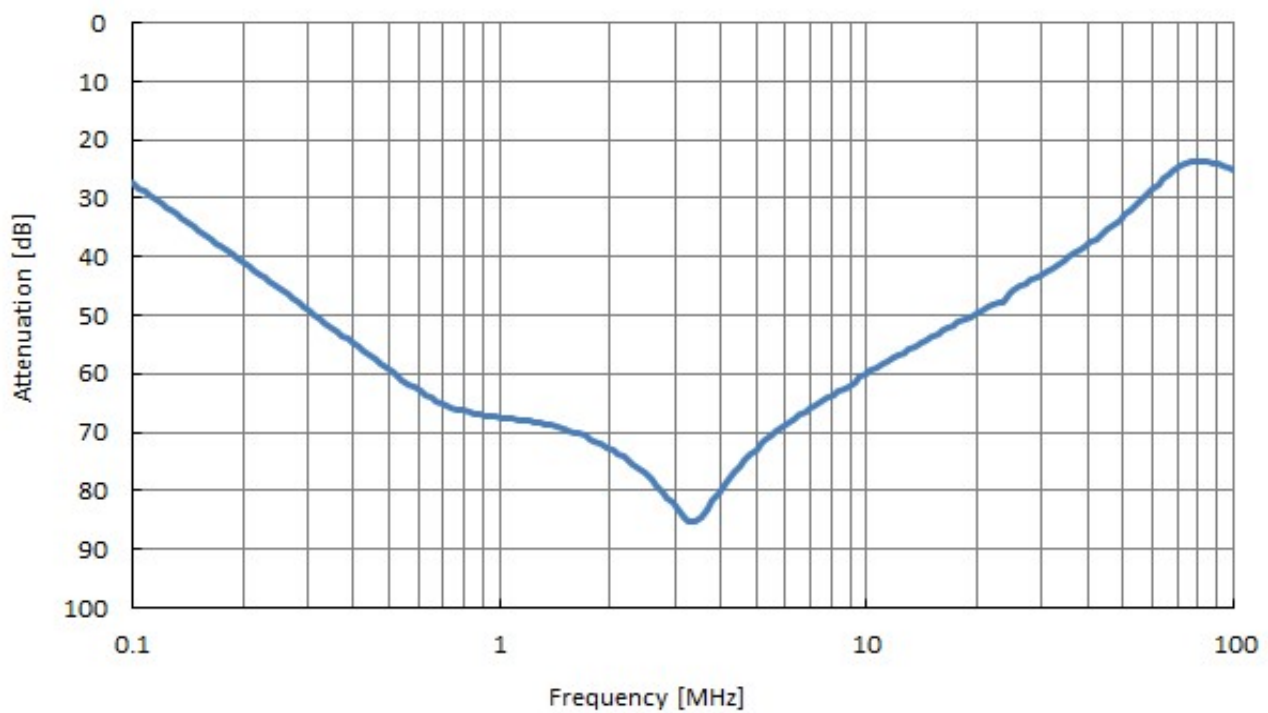
代表特性(30A)
