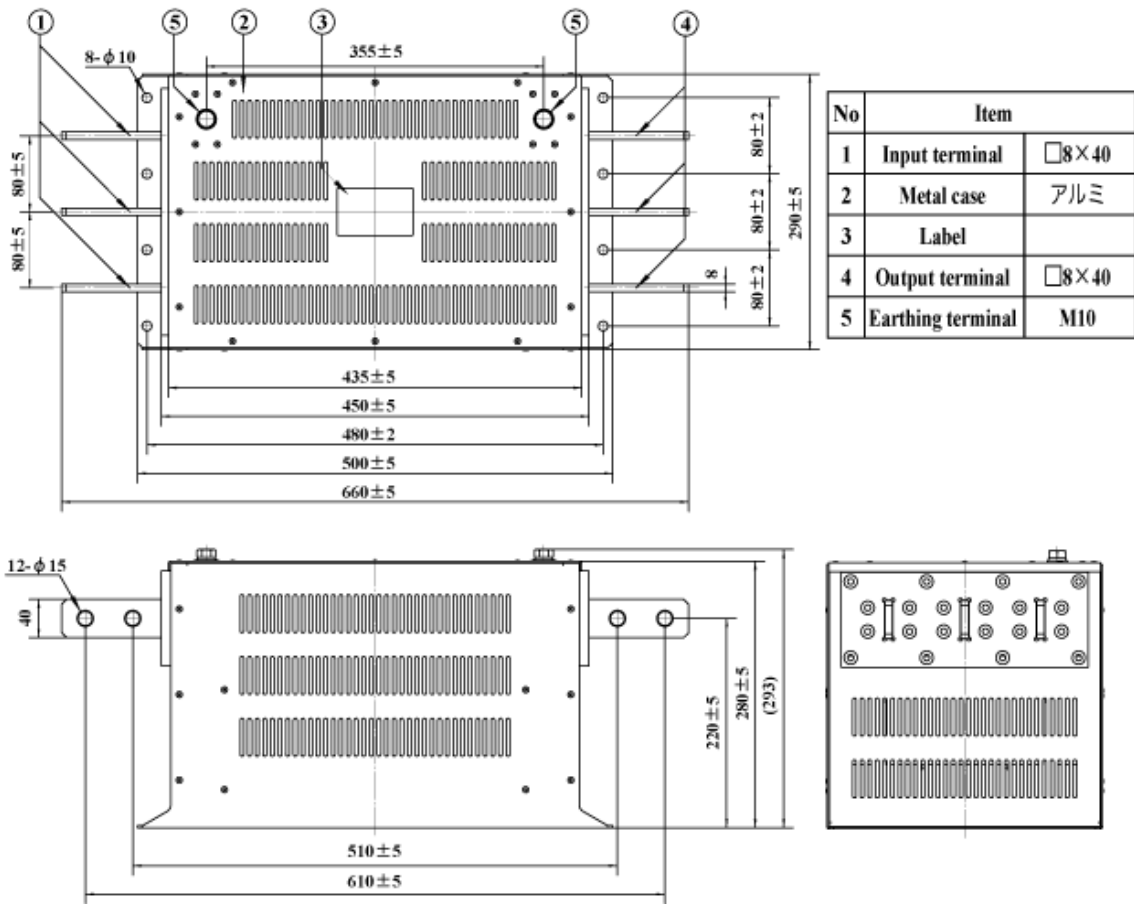
fig. 6 (900, 1000A)
