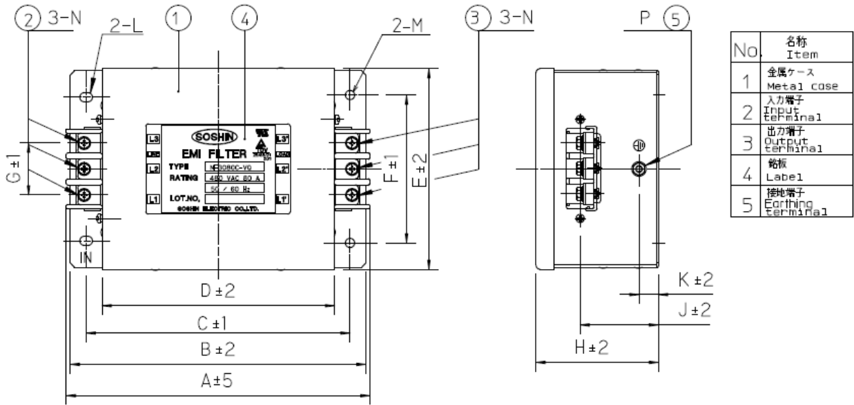
fig. 1 (50-150A)
