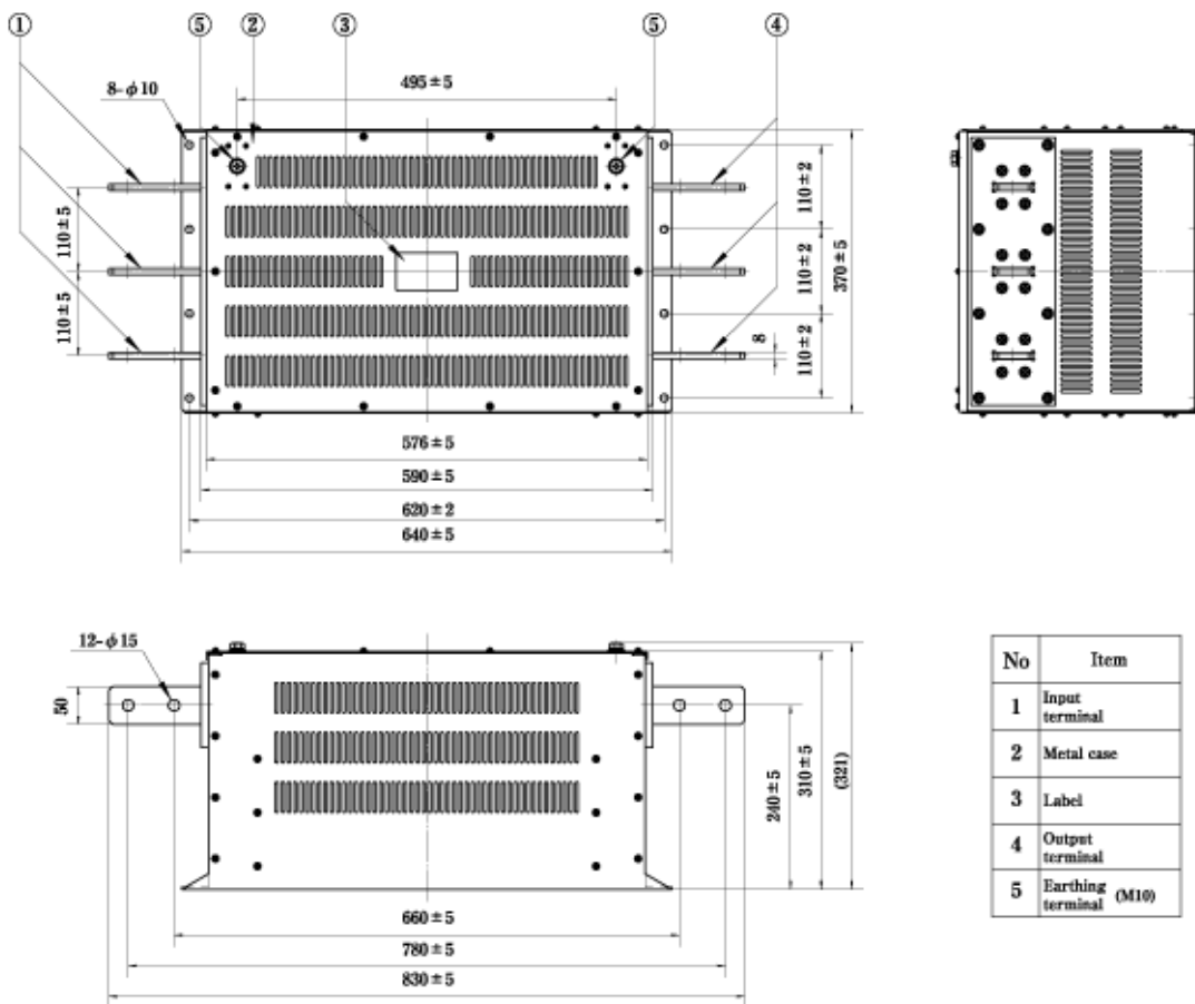
fig. 6 (900, 1000A)
