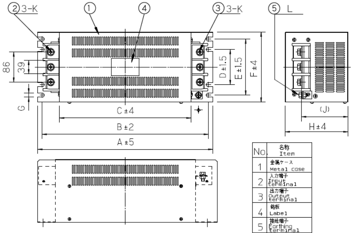
fig. 2 (200-350A)
