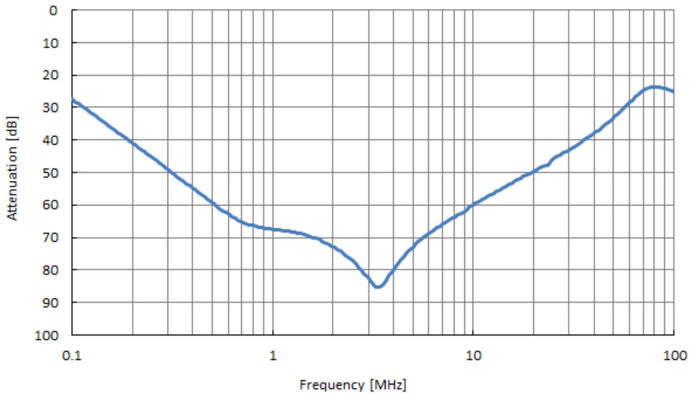
代表特性(30A)
